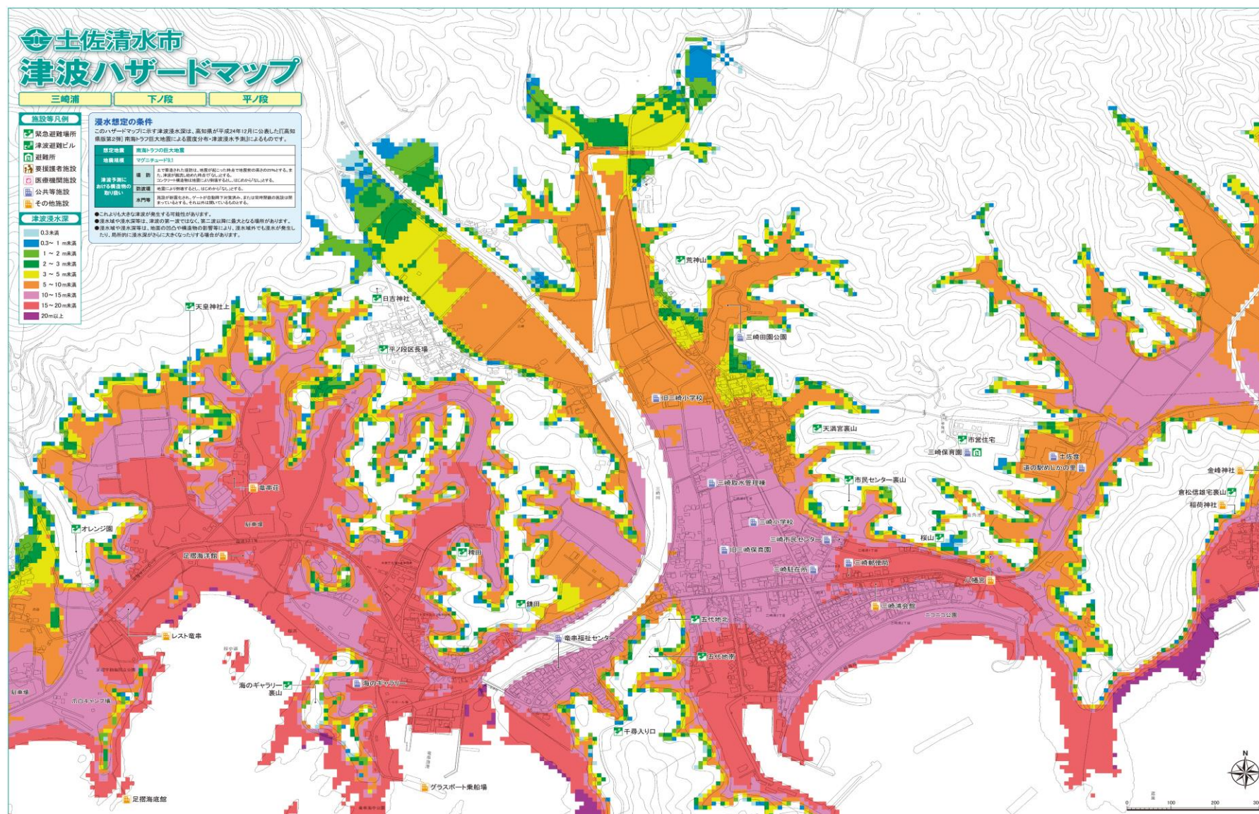
図 3.2 津波浸水予測図（下ノ段地区）
