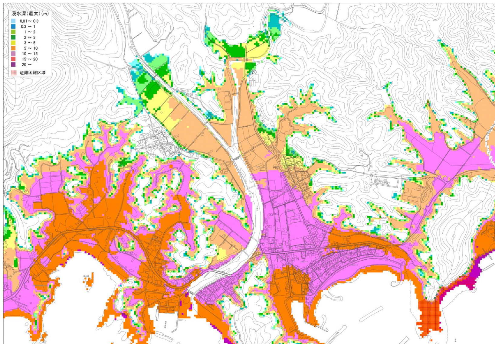
図 4.2 避難困難区域算定結果図（下ノ段地区）
