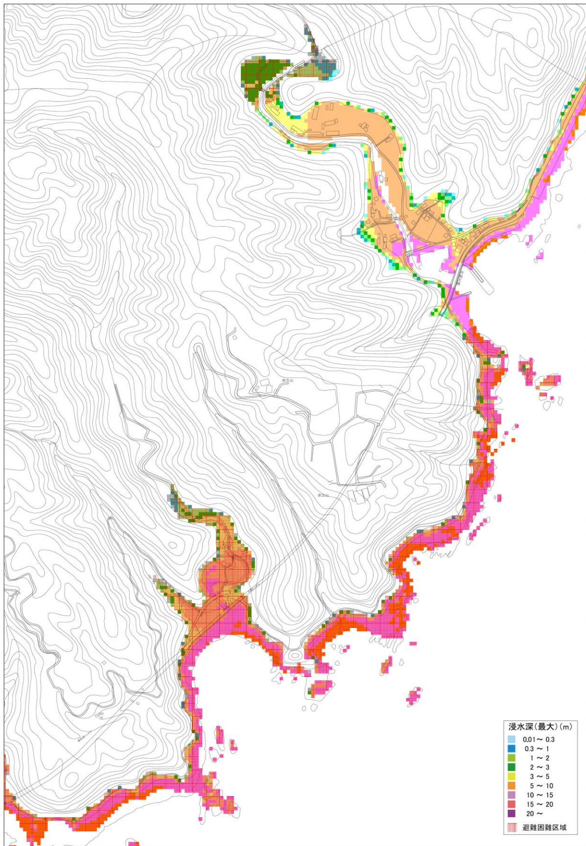
図 4.2 避難困難区域算定結果図（南朶ノ浦地区）
