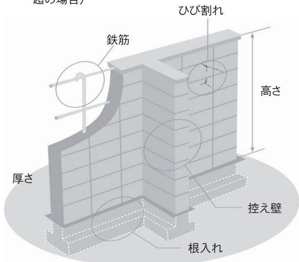
出典：パンフレット「地震からわが家を守ろう」 日本建築防災協会 2013.1より一部改
