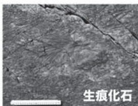
黒い部分 泥岩 白い部分 凝灰岩
